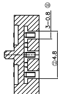
SEC A-A
