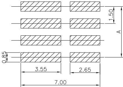
P.C.Board Layout
