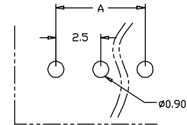
P.C.B LAYOT
